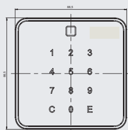
dormakaba Kompakteser 91 12 Front und Rückwand
